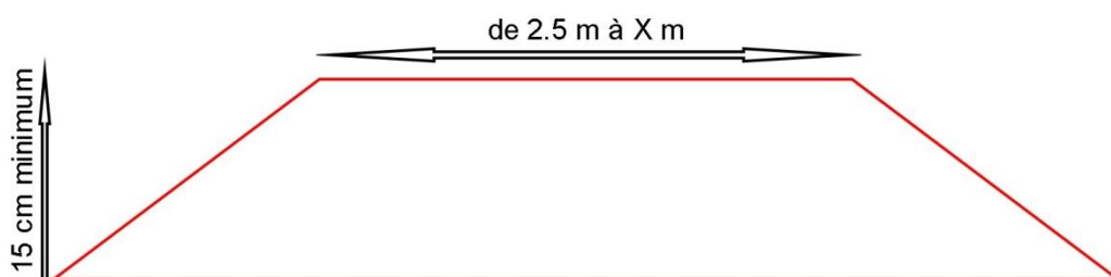
Ceci n'est pas un ralentisseur « trapézoïdal » mais un « plateau traversant » dont la forme n'est pas un « trapèze »
