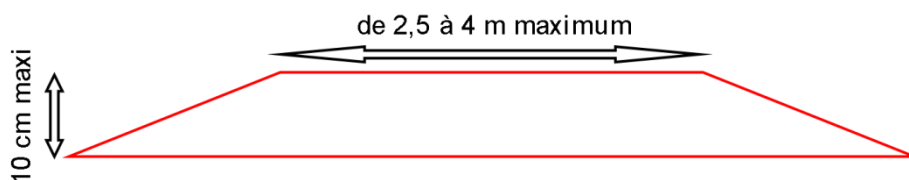
Le ralentisseur « trapézoïdal » tel que décrit dans la loi (décret 94-447 + norme NF 98-300)
